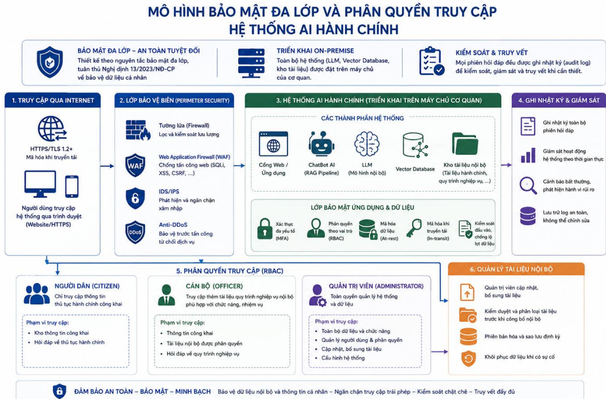
Hình 5: Mô hình bảo mật và phân quyền truy cập hệ thống
